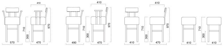
2093-1961 玄海 N スタンド椅子 1520 玄海ⅡN 背もたれ 1540×2 玄海 N アーム×2 張地：色舞 SH-12 (Bランク)
