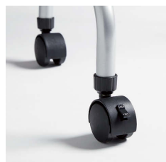
■アジャスト機能付キャスター テーブルの高さを微調整できます。
