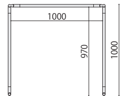
QSB説明(レイアウト寸法図)
