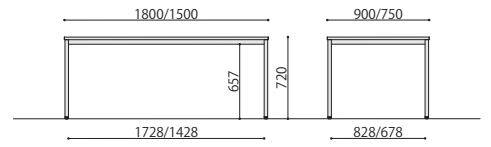
ASO-M1890/1575
