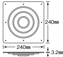
No.103 240×240 木ネジ8ヶ穴 ¥1,250
