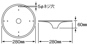
No.101 280mmφ ラッパ型十字穴 溶接用受座 38.1φ、42.7φパイプ用 ¥1,100
