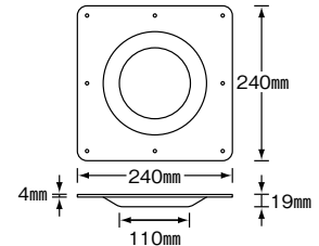
No.116・No.117 240×240 木ネジ8ヶ穴 No.116 ボルト式ノックダウン用受座 60.5φ、76.3φ、101.6φパイプ用 ¥2,050 No.117 溶接用受座 ¥1,350
