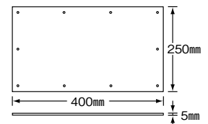
No.107 250×400 木ネジ10ヶ穴 ¥2,400
