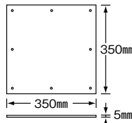
No.106 350×350 木ネジ8ヶ穴 ¥2,800
