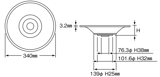
No.112 340mmφ ラッパ型6ヶ穴 ノックダウン受座 76.3φ、101.6φ(1.6t)、139φ(2t)パイプ用ボルト式、溶接可 ¥3,150
