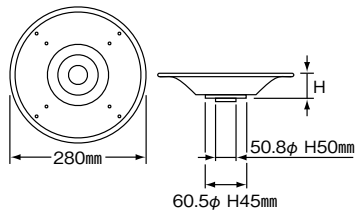
No.108 280mmφ ラッパ型十字穴 ノックダウン受座 50.8φ、60.5φ(1.6t)パイプ用ボルト式、溶接可 ¥2,100
